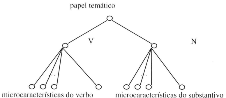
Figura 1. A arquitetura conexionista para um papel temático.
